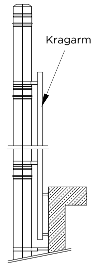
Bild 5-19: Aufbau mit Kragarm
