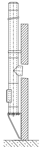
Bild 5-3: Aufbau Grundplatte mit Kondensatablauf und Konsolblech „schenkelabwärts“
