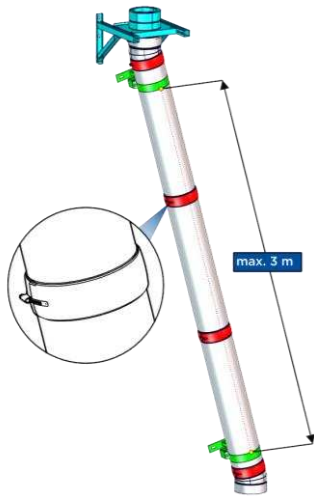
Bild 5-23: Schrägführung 15°
