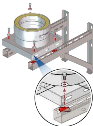
Bild 5-6 Grundplatte auf Wandstützen & Querträger montiert
