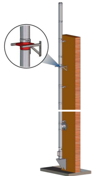
Bild 5-21: Aufbau mit Grundplatte für Zwischenstütze
