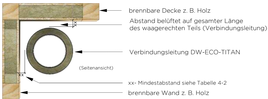
Bild 4-2: Einbau als Verbindungsleitung bis T600
