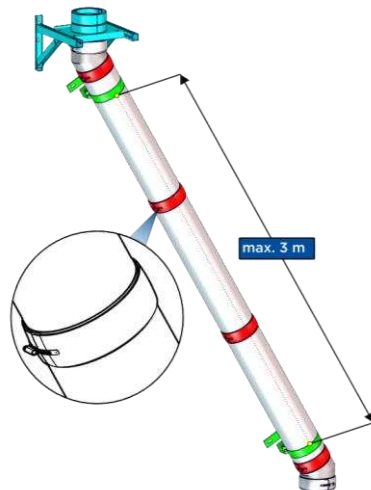
Bild 5-24: Schrägführung 30°
